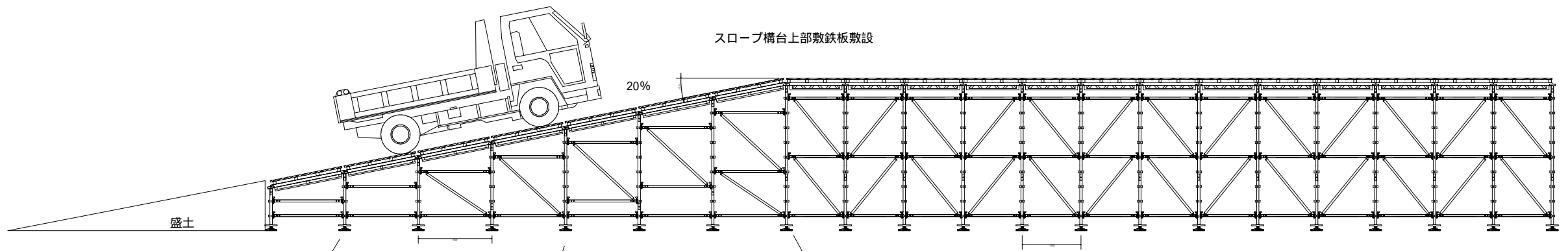
構台 (15.6m) 断面図
