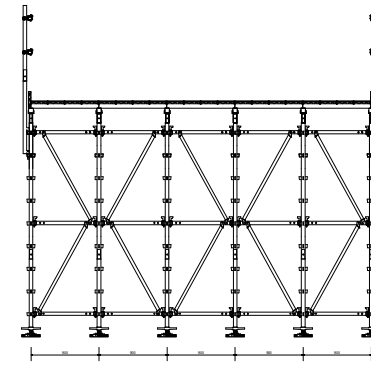
構台 (15.6m) 断面図
